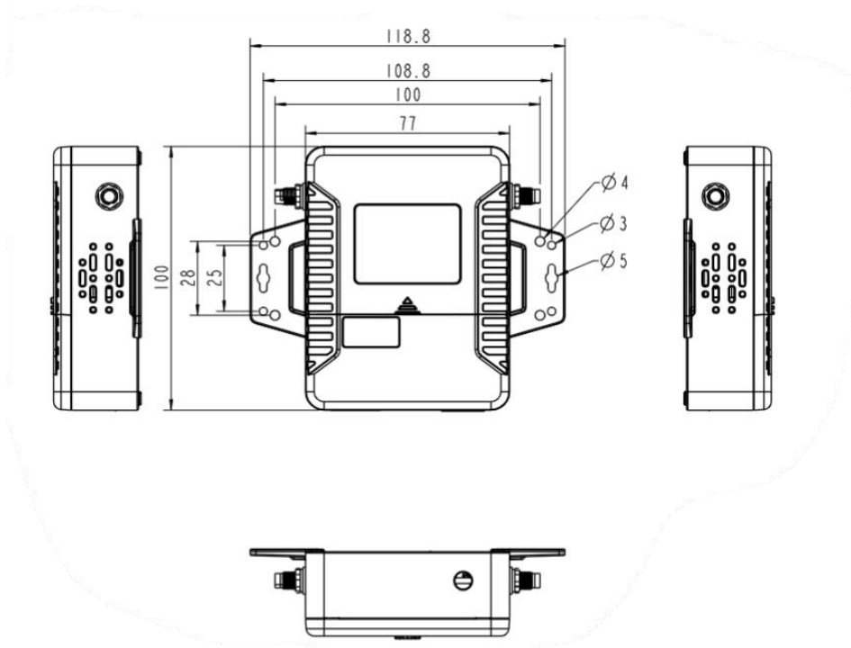
图 4-1 外观尺寸图
