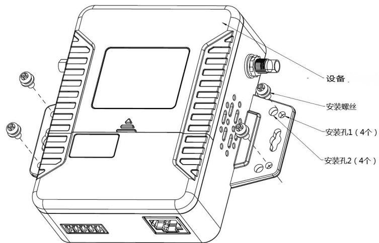
图 4-4 产品安装示意图
