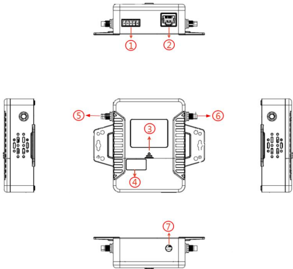
图 4-2 接口编号图
