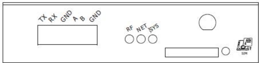
图 4-1 指示灯面板图
