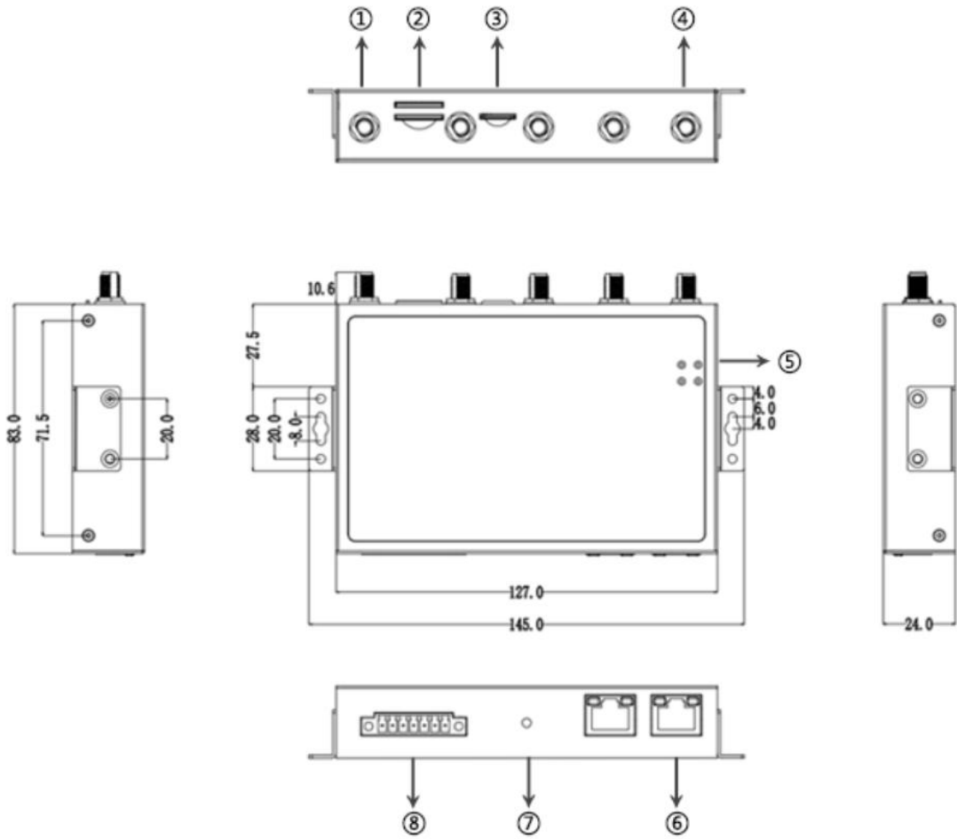
图 3-1 接口尺寸图
