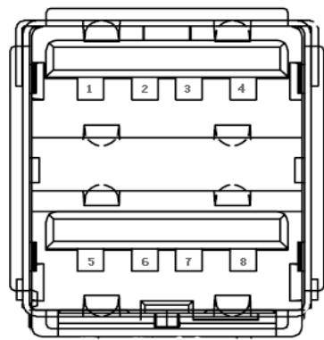
图：双层 USB 接口图
