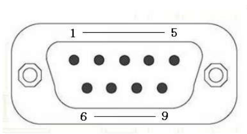
图 3-4-1： RS-232 接口图
