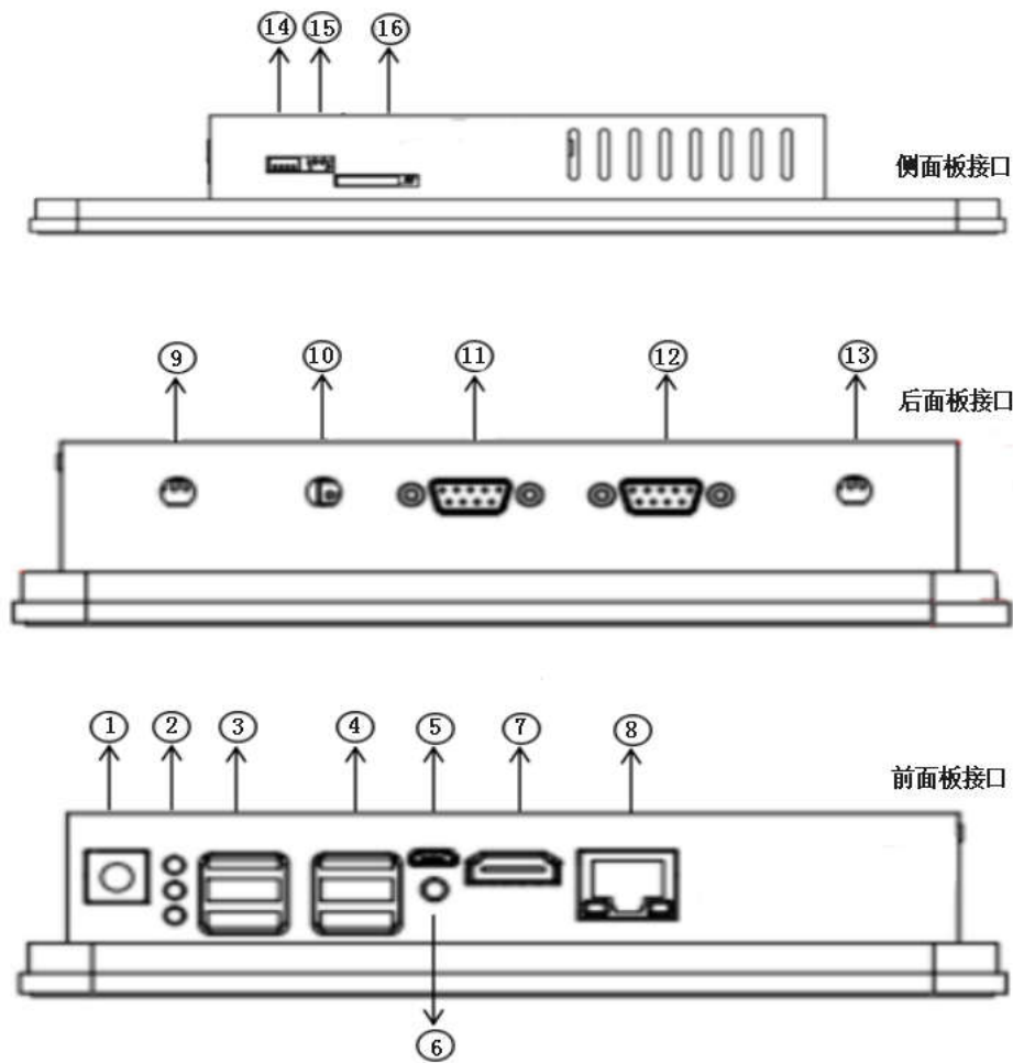
图 3-2-1 侧面板接口表
