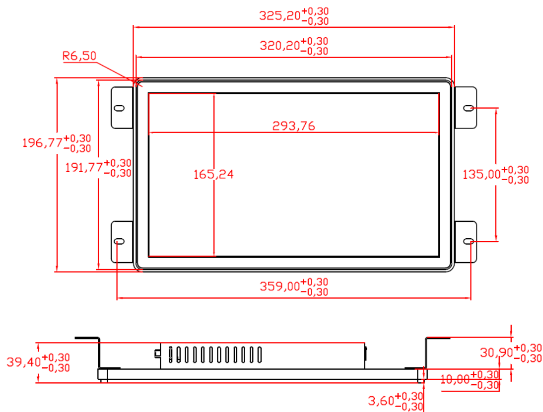
图 3-1 一体机结构尺寸图
